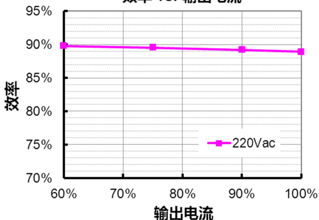
EBV-150S048SV 效率 vs. 输出电流
