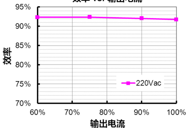
EBV-200S012SV 效率 vs. 输出电流
