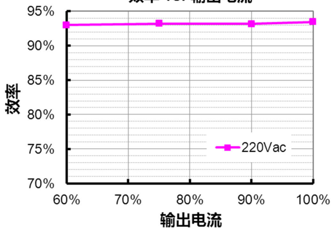
EBV-200S048SV 效率 vs. 输出电流
