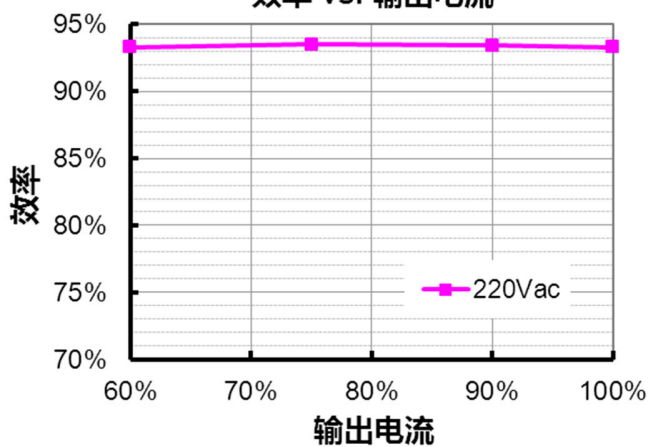
EBV-200S024SV 效率 vs. 输出电流
